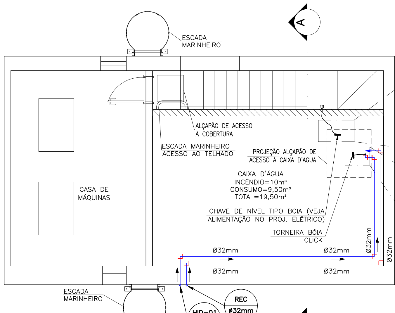
PROJETO HIDRÁULICO PLANTA DA CAIXA D'ÁGUA ESC: 1:50
