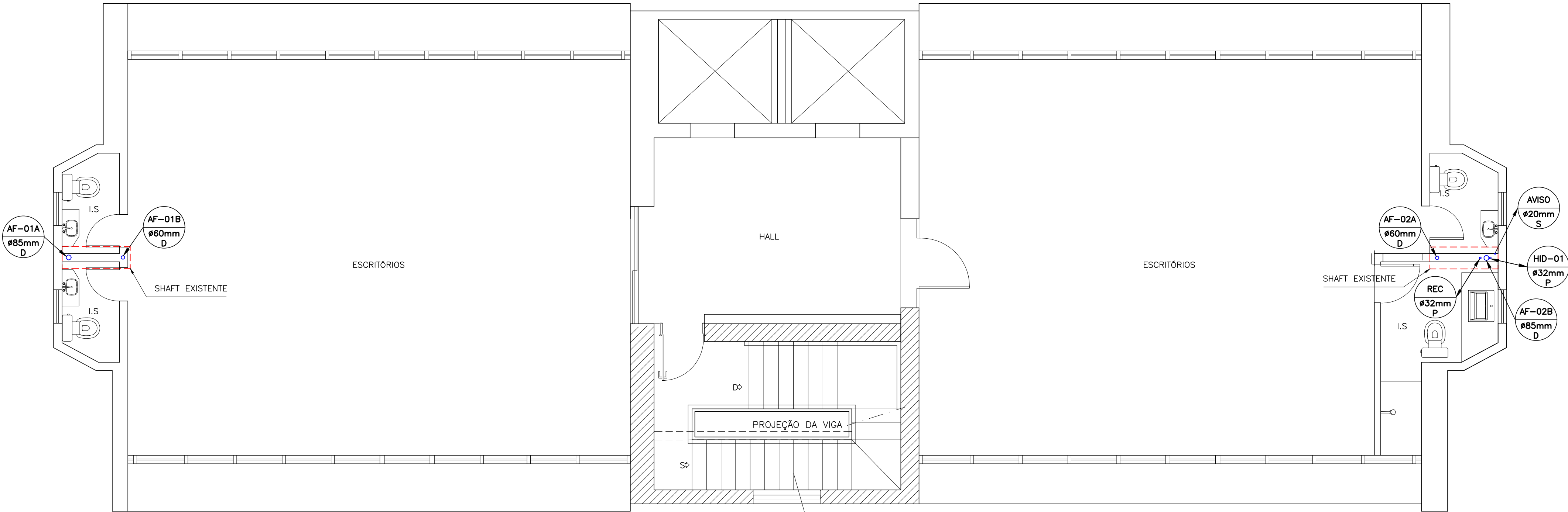
PROJETO HIDRÁULICO PLANTA PVTO TIPO ESC: 1:50
