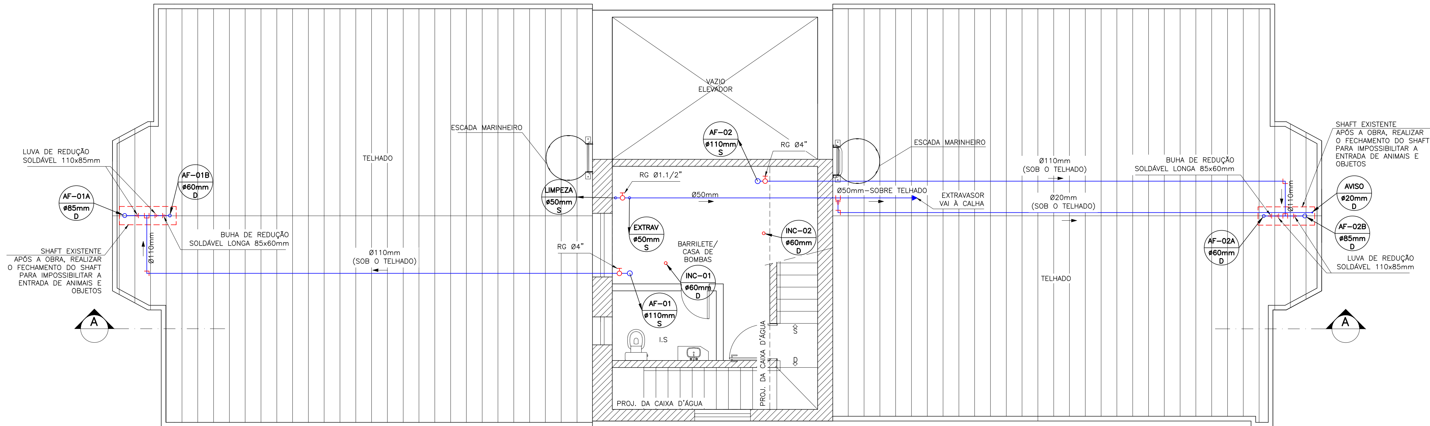
PROJETO HIDRÁULICO BARRILETE — DISTRIBUIÇÃO ESC: 1:50
